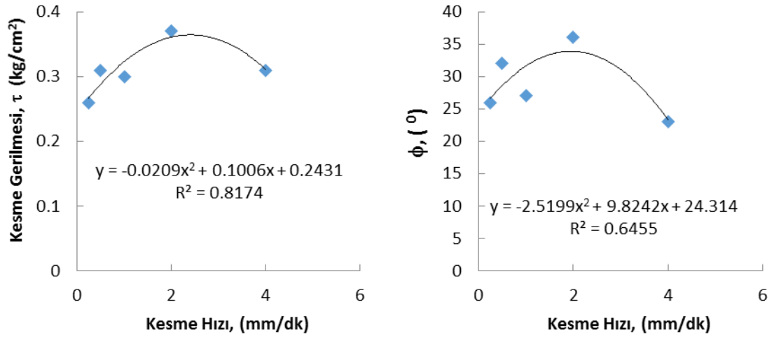
Şekil.5 Doygun kum örnekleri için kesme hızı-içsel sürtünme açısı eğrisi (Shearing speed-internal friction angle curve for saturated sand samples)
