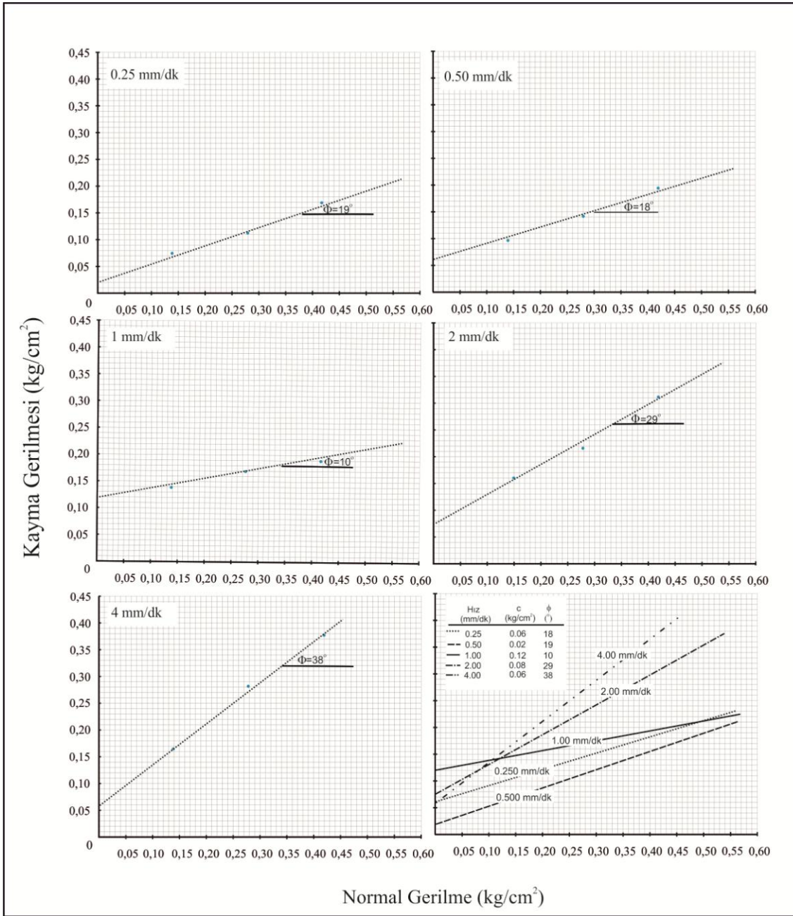
Şekil 4. Doygun olmayan (kuru) ortamda yapılan kesme kutusu deneyine ait normal gerilme-kesme gerilme grafikleri (Normal stress - shear stress graphs of unsaturated (dry) condition belong to shear box test)
