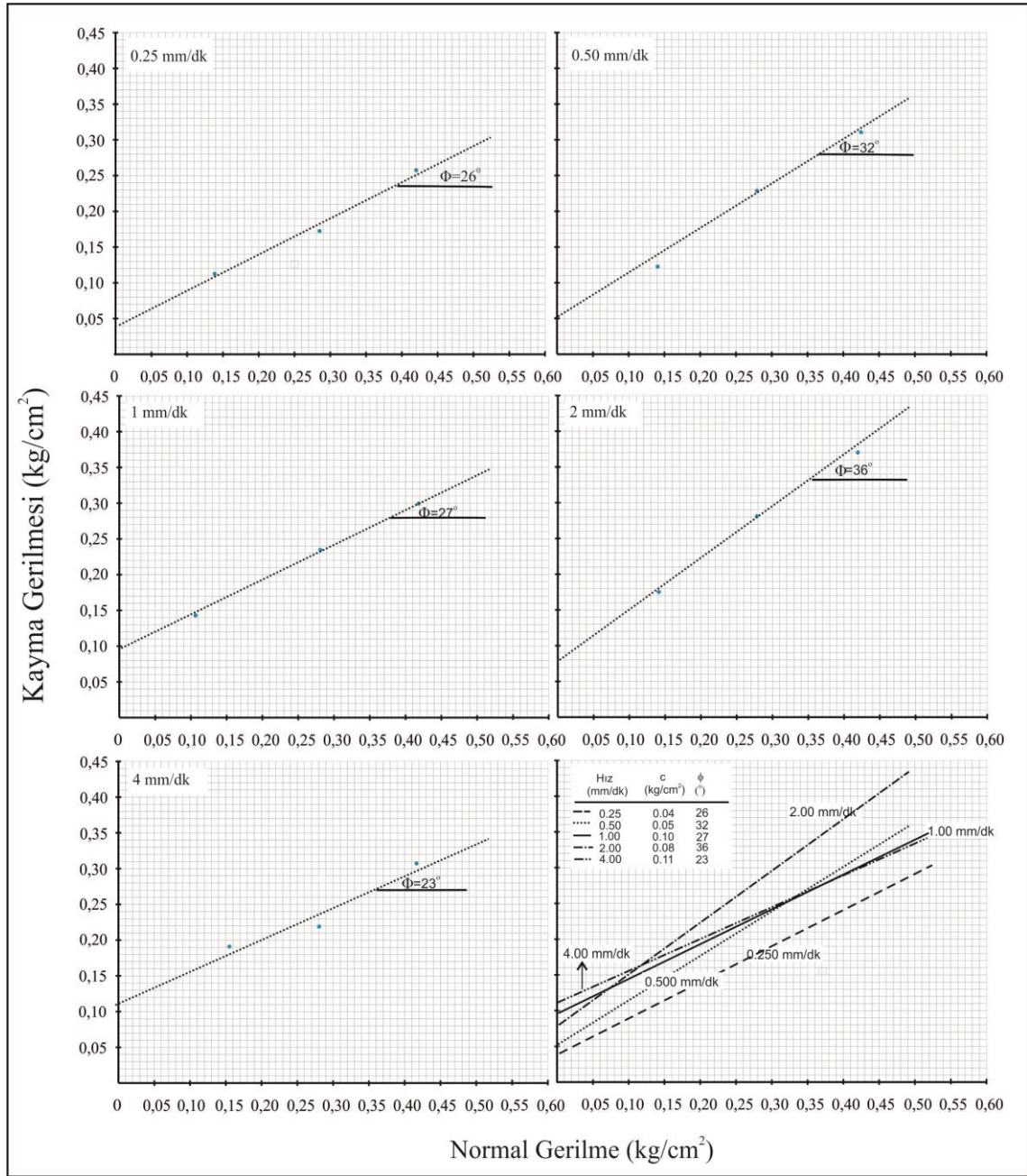
Şekil 3. Doygun ortamda yapılan kesme kutusu deneyine ait normal gerilme-kesme gerilme grafikleri (Normal stress - shear stress graphs of saturated condition belong to shear box test)
