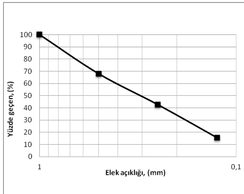
Şekil.2 Numunenin tane boyu dağılım grafiği (Graph of sample grain size distribution).
