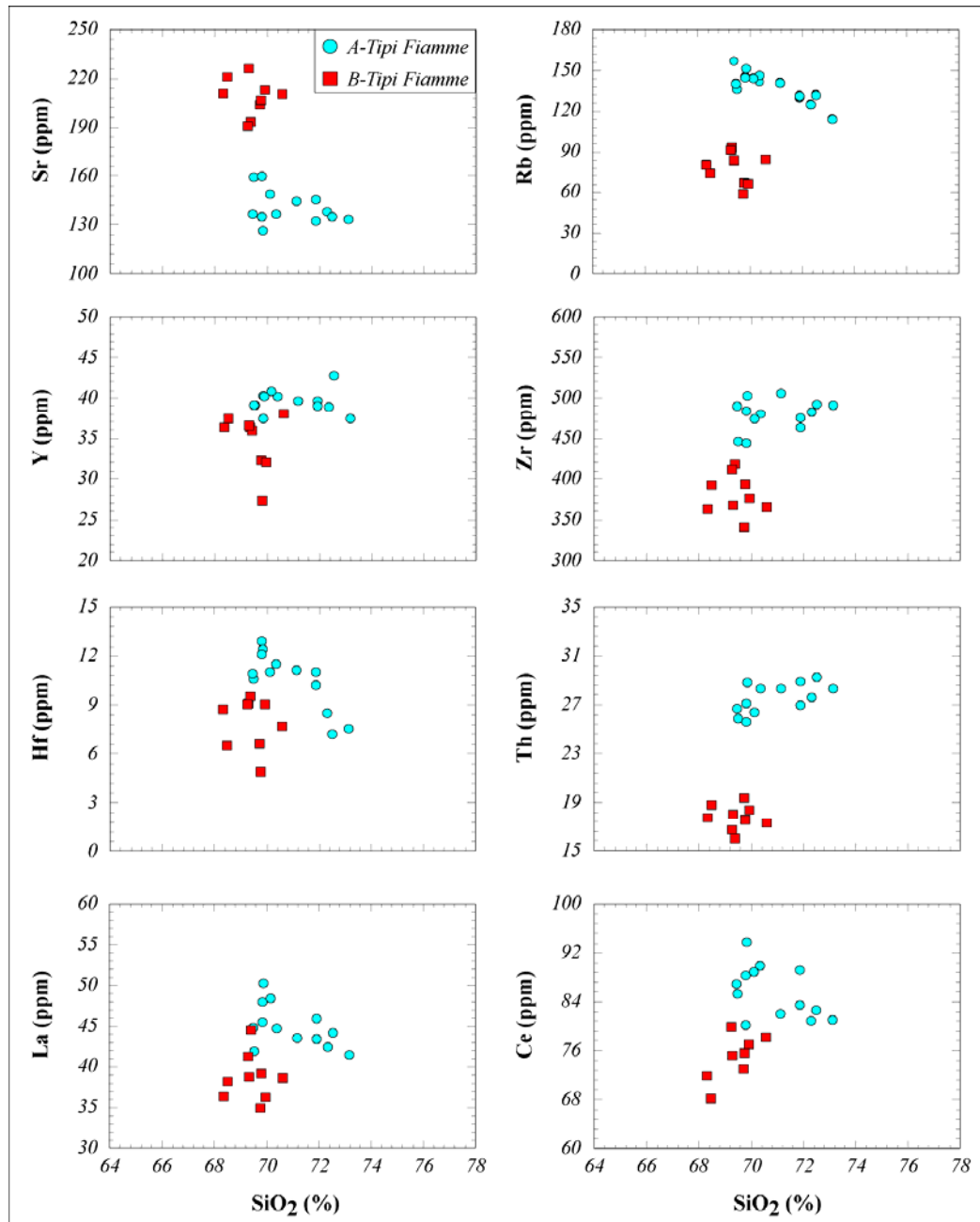
Şekil 7. A ve B tipi fiamme örneklerinin SiO 2 (wt.%) - iz element(ppm) değişim diyagramları. Figure 7. SiO 2 (wt.%) versus trace elements (ppm) variation diagrams for the A and B type fiamme.
