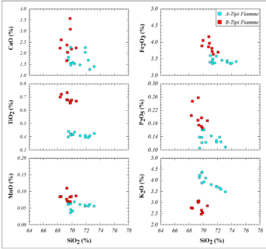
Şekil 6. Ave B tipi fiamme örneklerinin \text{SiO}_2(\%) -ana oksit element(%) değişim diyagramları.
