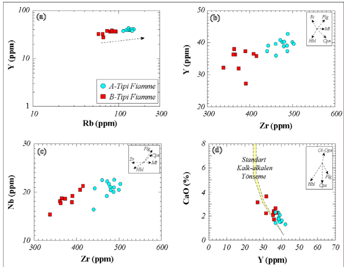
Şekil 10. A ve B tipi fiamme örneklerinin a) logRb(ppm)-logY(ppm) (Pearce ve diğ., 1990) b) Zr(ppm)-Y(ppm) ve c) Zr(ppm)-Nb(ppm) (Pearce ve Norry, 1979) d) Y(ppm)-CaO(wt.%) diyagramları (Lambert ve Holland, 1974) (kesikli çizgilerle gösterilen vektörler minerallerin fraksiyonlaşma yönlerini göstermektedir).
