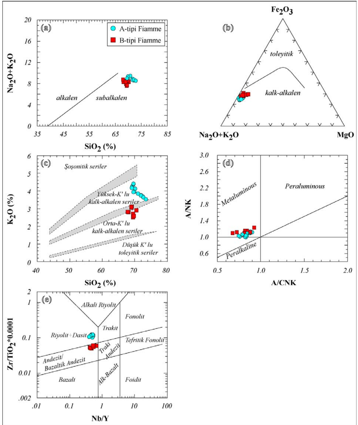
Şekil 5. A ve B tipi fiamme örneklerinin a) \text{SiO}_2(\%) - \text{Na}_2\text{O}+\text{K}_2\text{O}(\%) (Le Maitre ve diğ., 1989) b) AFM (toleyitik-kalkalkalen ayırım çizgisi Irvine ve Baragar 1971' e göre) c) \text{SiO}_2(\%) - \text{K}_2\text{O}(\%) (Le Maitre ve diğ., 1989) d) \text{A/NK} - \text{A/CNK} (Maniar ve Piccoli, 1989) e) \text{Nb/Y} - \text{Zr}/\text{TiO}_2 \cdot 0.0001 diyagramlarındaki konumları.
