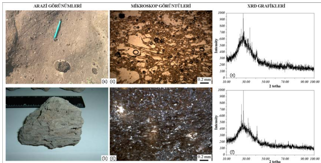
Şekil 3. A-tipi fiamme örneklerinin a, b) arazi ve yakından görünümüleri c, d) mikroskop görüntüleri e, f) XRD grafikleri.
