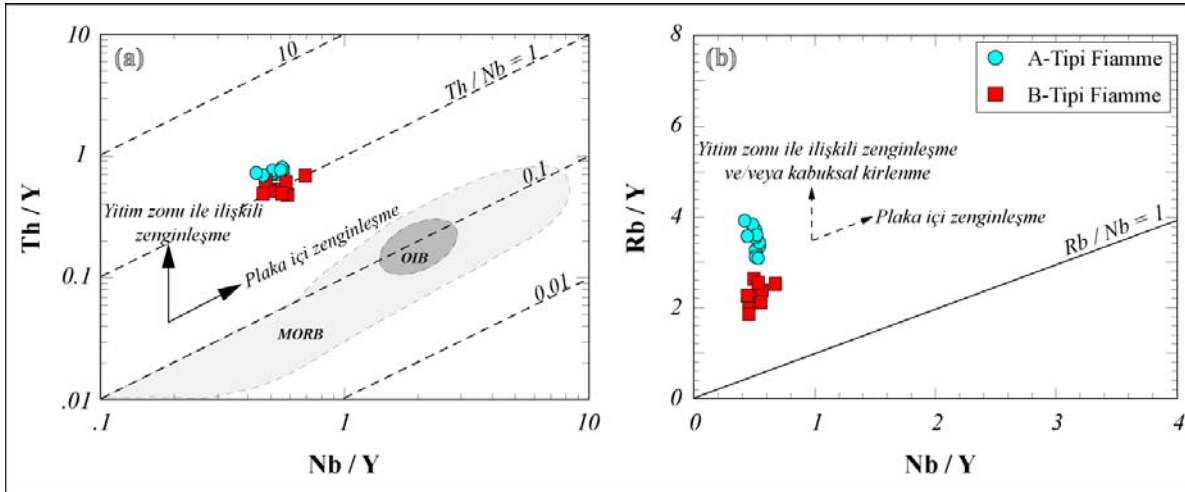
Şekil 11. A ve B tipi fiamme örneklerinin a) \log \text{Nb}/\text{Y} karşı \log \text{Th}/\text{Y} (Pearce, 1983) ve b) \text{Nb}/\text{Y} karşı \text{Rb}/\text{Y} (Edwards ve diğ., 1991) değişim diyagramları.
