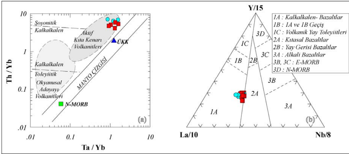
Şekil 12. A ve B tipi fiammelerin a) logTh/Yb karşı logTa/Yb diyagramındaki konumları (Pearce, 1983; ortalama N-MORB (Pearce, 1983) ve Üst Kıta Kabuğu değerleri (Rudnic ve Gao, 2004) karşılaştırma için kullanılmıştır) b) Y/15-La/10-Nb/8 üçgen diyagramındaki konumları (Cabanis ve Lecolle, 1989).
