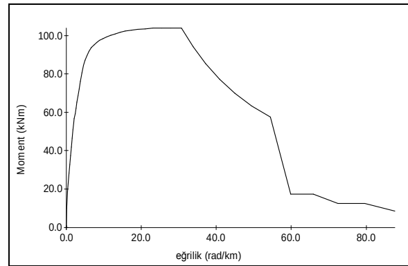
Şekil 12. Response2000'e göre TİP C deney elemanı teorik moment-eğrilik diyagramları.
