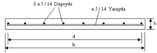
a) TİP A deney elemanlarına ait donatı düzenleri.
