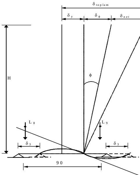
Şekil 8. Net yatay deplasmanların hesaplanması (ölçüler cm'dir). Figure 8.
