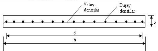
b) TİP B deney elemanlarına ait donatı düzenleri.
