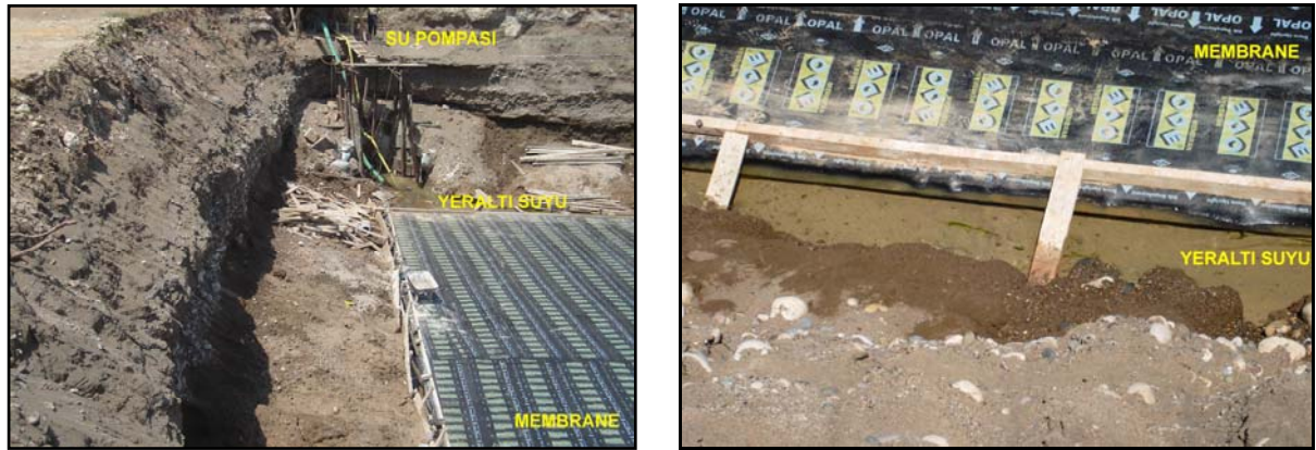
Şekil 7. Yüzeye oldukça yakın seviyede yeraltı suyunun olduğu bir yüzey kazısı.
