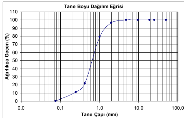
Şekil 3. Kum çökellerine ait tipik tane boyu dağılım eğrileri.
