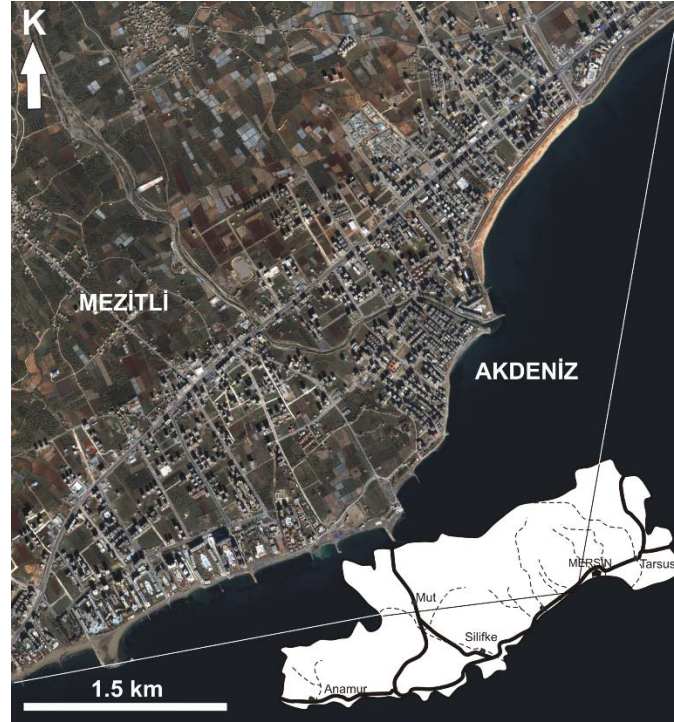
Şekil 1. İnceleme alanının Mersin ili yerleşim alanı içerisindeki yerini gösteren lokasyon haritası.
