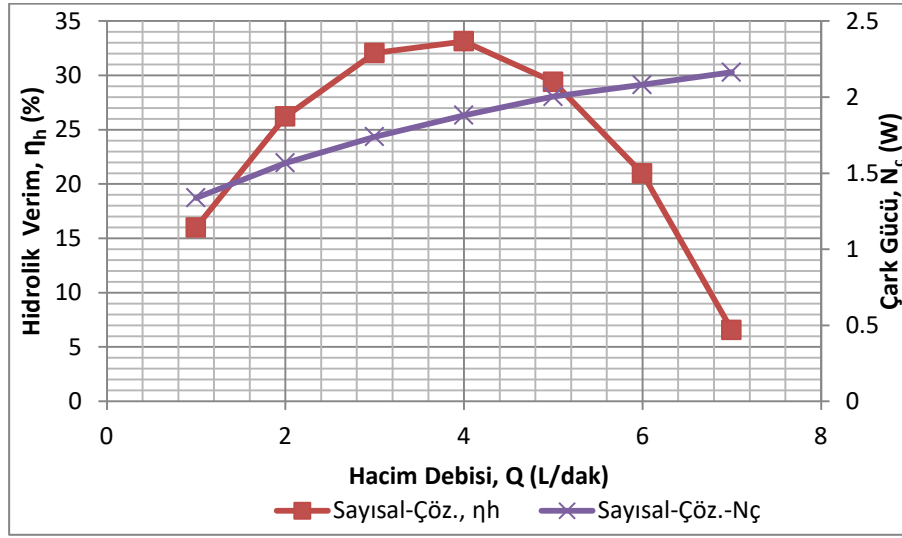
Şekil 10.b Su-gliserin çözeltisi için sayısal hidrolik verim ve çark gücü grafiği
