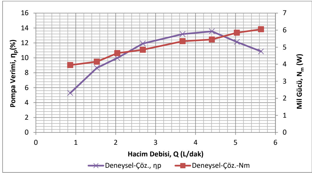
Şekil 9.b Su-gliserin çözeltisi için deneysel güç ve verim grafiği
