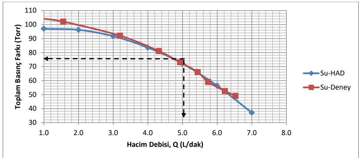
Şekil 5. Deneysel sonuçların HAD sonuçlarıyla karşılaştırılması
