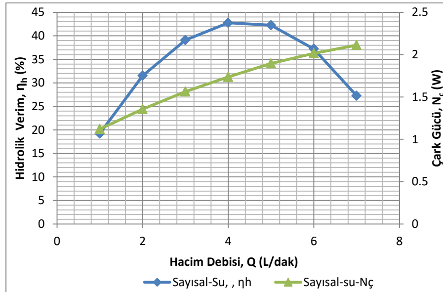
Şekil 10.a Su için sayısal çark gücü ve hidrolik verim grafiği
