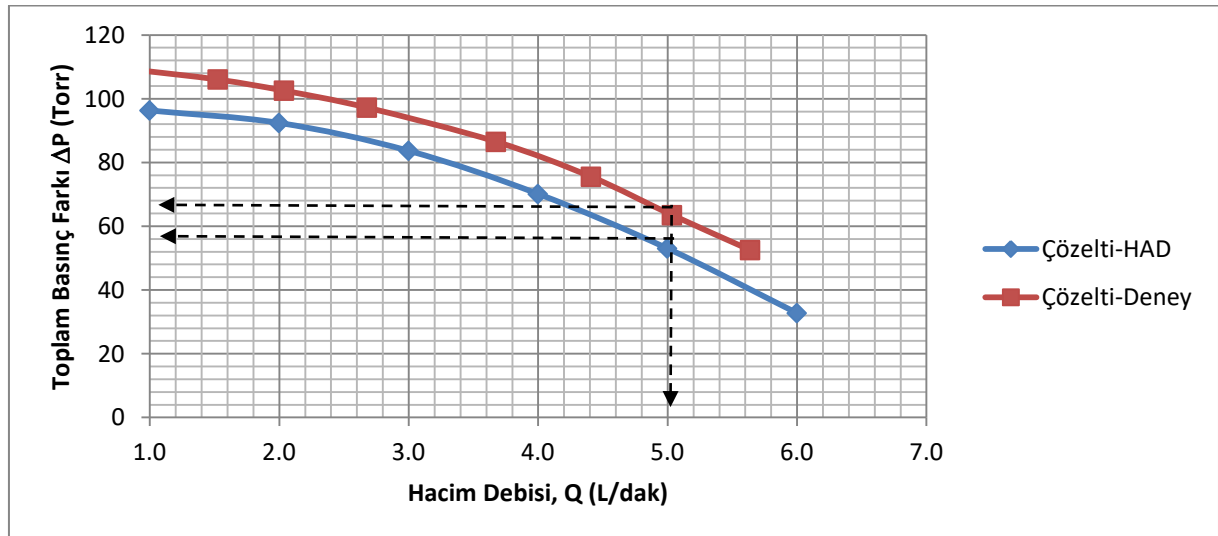
Şekil 7. Deneysel sonuçlarının HAD simülasyon sonuçlarıyla karşılaştırılması
