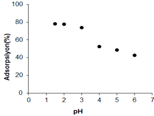
Şekil 6. (Kts/Kao) boncuklarıyla Cr(VI) adsorpsiyonuna pH'ın etkisi (Adsorpsiyon şartları: Cr(VI) konsantrasyonu, 10^{-3} mol/L; adsorbent dozu, 2g/L; temas süresi, 2 saat; sıcaklık, 25 \pm 1 °C). Figure 6. Effect of pH on the adsorption of Cr(VI) by (Kts/Kao) beads. (Adsorption conditions: concentration of Cr(VI), 10^{-3} mol/L; adsorbent dosage, 2g/L; contact time, 2 h; temperature, 25 \pm 1 °C).
