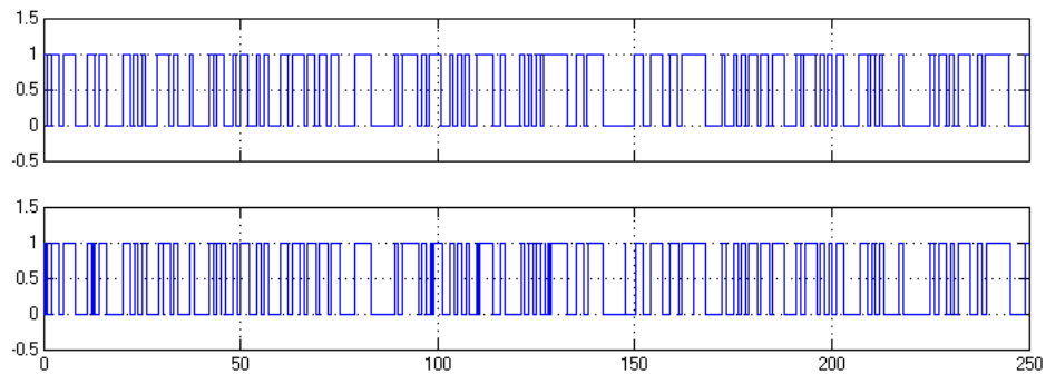
Şekil 12. a) İletilen bilgi sinyali b) HSA tabanlı alıcıda elde edilen bilgi sinyali.
