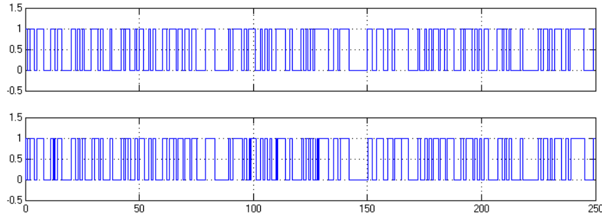
Şekil 14. a) İletilen bilgi sinyali b) HSA tabanlı FPGA alıcıda elde edilen bilgi sinyali.
