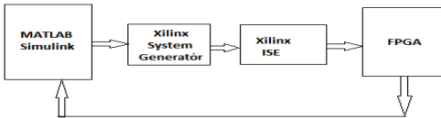
Şekil 5. FPGA tabanlı Xilinx System Generator ile hardware Co-simulation.
