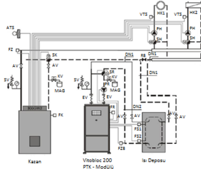
Şekil 8. Kurgulanan ısı depolu PTKM sistem şeması (Viessmann Vitobloc 200 PTK)
