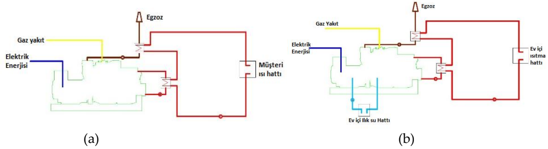
Şekil 5 a. Ceket suyu sıcaklığı ve egzoz ısı geri kazanımı, b. Intercooler ısı geri kazanımı
