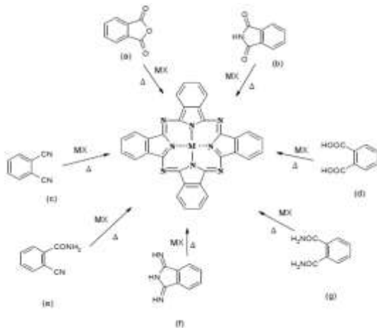
Şekil 2. Ftalosiyanın için genel sentez şeması.
