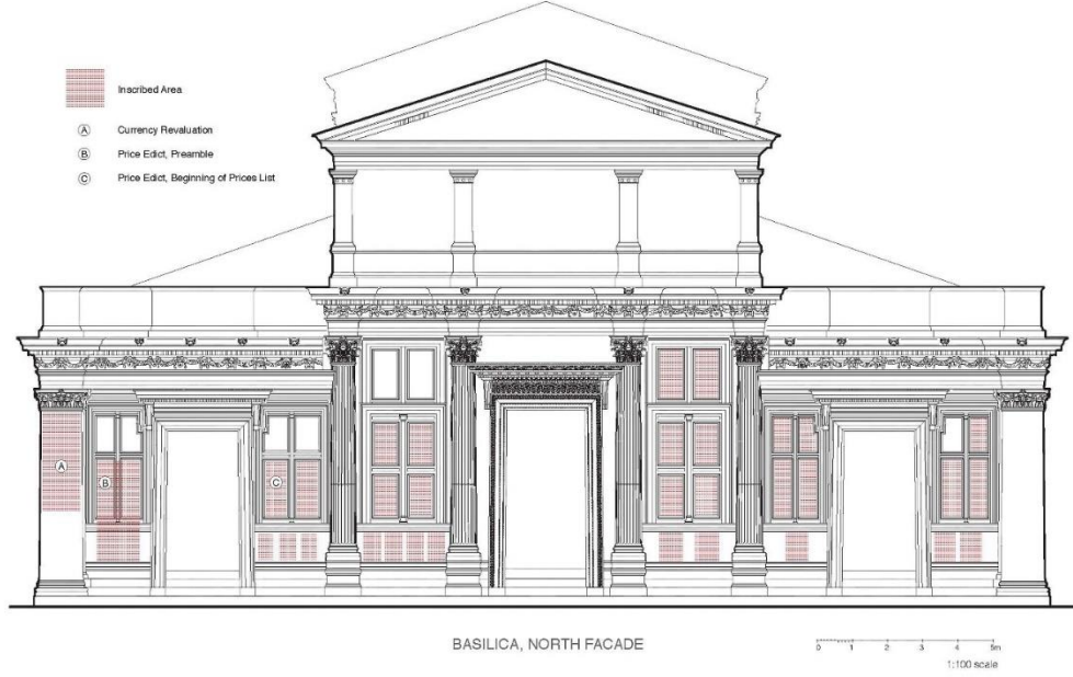
Fig. 15. Bazilika, ön (kuzey) cephe rekonstrüksiyon çizimi
