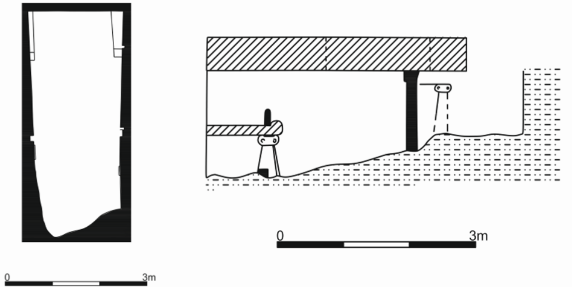
Fig. 11. ALN.20.KN.M57 Numaralı Oda Mezar, Çizimi
