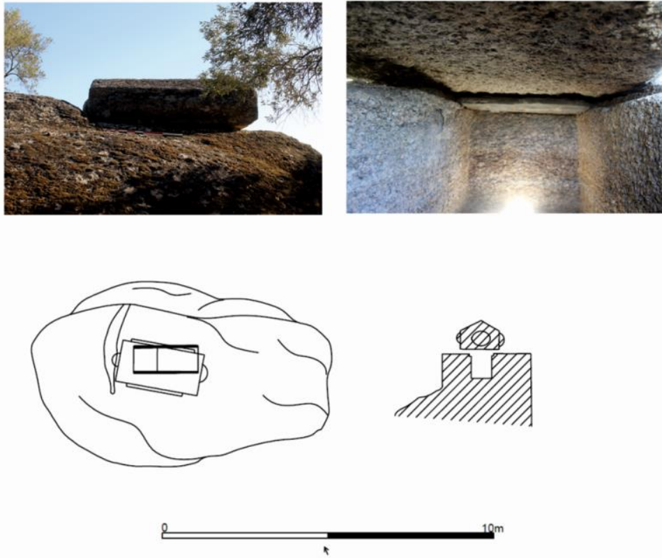
Fig. 15. ALN.21.KN.KH.10 Numaralı Khamosorion Mezar Çizimi
