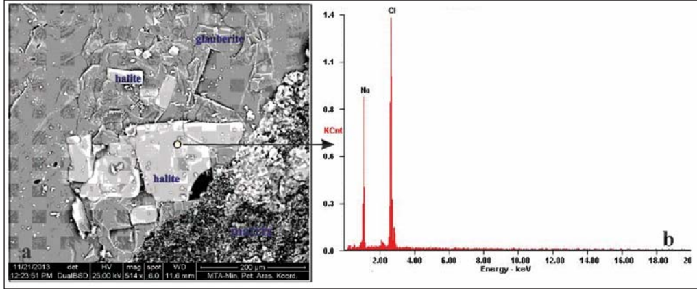
Şekil 27- Glauberit minerali üzerinde gelişmiş prizmatik özşekilli halit kristalleri, (O: kristal üzerinde alınan EDS analiz ölçüm noktası). (Yenidoğan-2 366,10 m XRD şekil 19).
