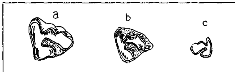
Fig. 2 - Comparaison des P_3 inferieures d' Alloptox . a) A. anatoliensis n. sp., holotype, AKÇ. 1, \times 10 b) A. gobiensis , \times 7,2 (Dawson, 1961). c) O. gobiensis , \times 5 (Young, 1932).
