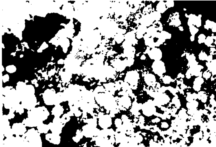
Foto 5 - Okular: 10, Objektiv: 25, im Immersionsöl. Das Kisa Bekir-Vorkommen in Ergani Maden. Pyrit (weiss) zeigt mit Kupferkies (von dunklerer Farbe) in Form von Kügelchen kolloidale Verwachsung. Sphalerit (grau), Gangminerale (schwarz) sind sichtbar.
