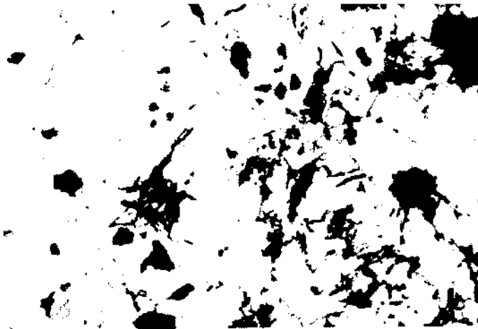
Foto 12 - Okular: 10, Objektiv: 16, im Öl. Das Kisa Bekir-Vorkommen in Ergani Maden. Im Pyrrhotin (hellgrau) Co-Pentlandit (in der Mitte und weiss). Kupferkies (von hellerer Farbe als Pyrrhotin), Pyrit (Relief aufweisend), Sphalerit (dunkelgrau) und Gang (schwarz).
