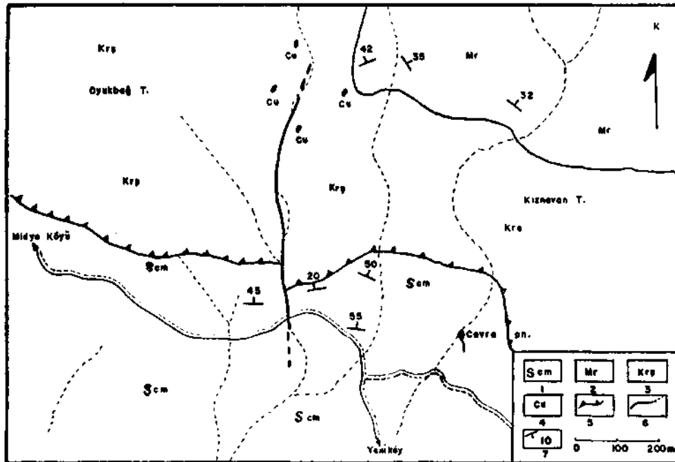
Abb. 5 - Geologische Karte des Gebiets von Diyarbakır-Çüngüş-Kayıslidere (Üzeyir Kesi).
