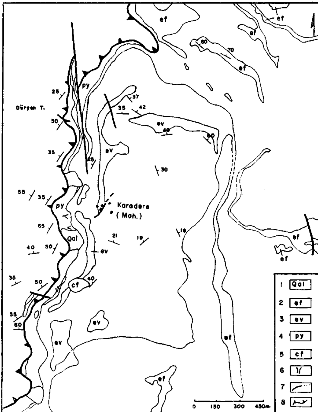
Abb. 4 - Geologische Karte des Kupfererzvorkommens in der Umgebung von Lıce-Karadere-Yayla (Hanefi Polat). 1 - Alluvion und Hangschutt; 2 - Flysch; 3 - Spilit, Diabas; 4 - Pyrat; 5 - Schlacke; 6 - Schurf; 7 - Verwerfung; 8 - Überschiebung.
