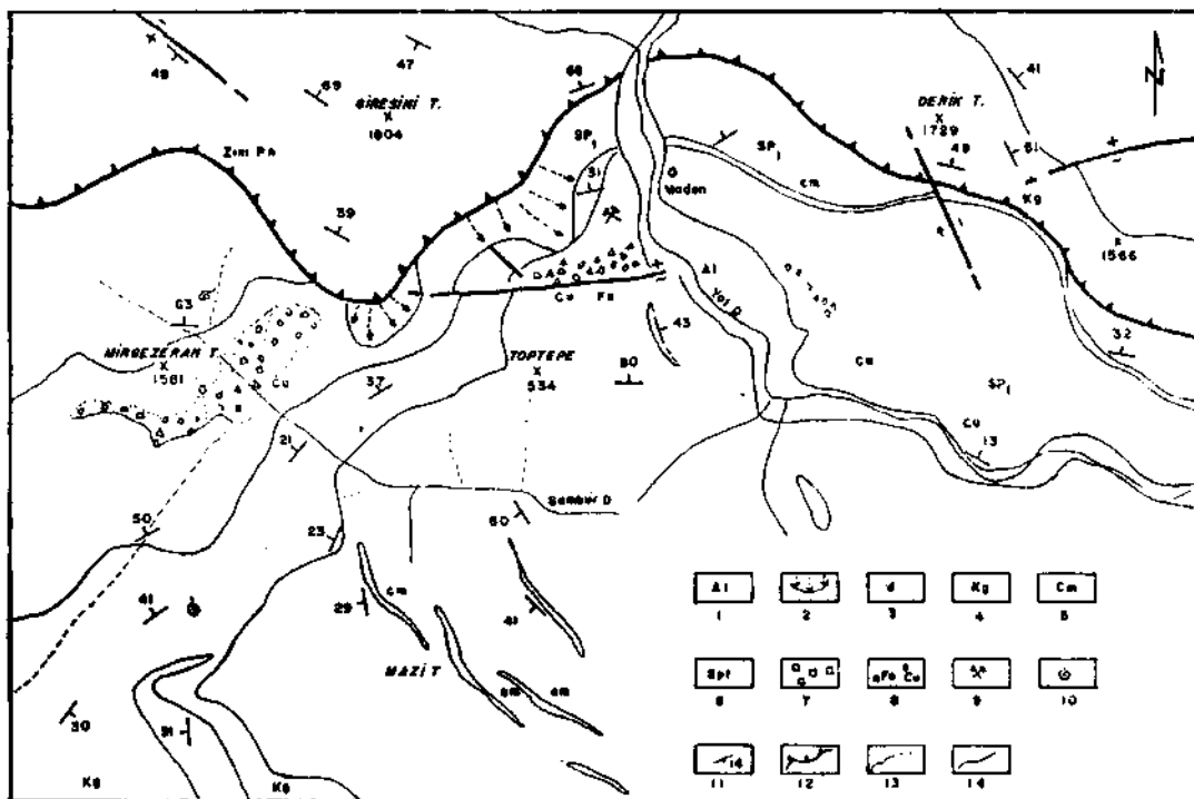
Abb. 3 - Geologische Karté der Umgebung von Siirt-Madenköy (Rüstem Yıldırım, Fahrettin Alyamaç, 1976). 1 - Alluvion; 2 - Kalksteindetritus; 3 - Dazit; 4 - Schotter; 5 - Schlammstein; 6 - Spilit. Diabas; 7 - Alteration; 8 - Kupfer- und Eisenmineralisation; 9 - Altes Bergwerk; 10 - Fossilfund- punkt; 11 - Schichtstreichen und -einfallen; 12 - Überschiebung; 13 - Verwerfung; 14 - Formation.
