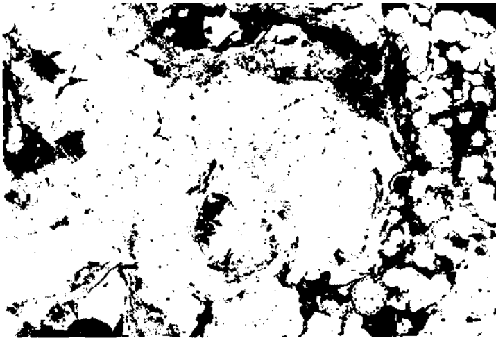
Foto 20 - Okular: 10, Objektiv: 25, im Immersionsöl. Die Lagerstätte von Siirt-Madenköy. Pyrit (hellstgrau) ist teils in Form von Kügelchen und teils zeigt er mit Kupferkies (hellgrau) kolloidale Verwachsung. Gangminerale und Löcher (schwarz).
