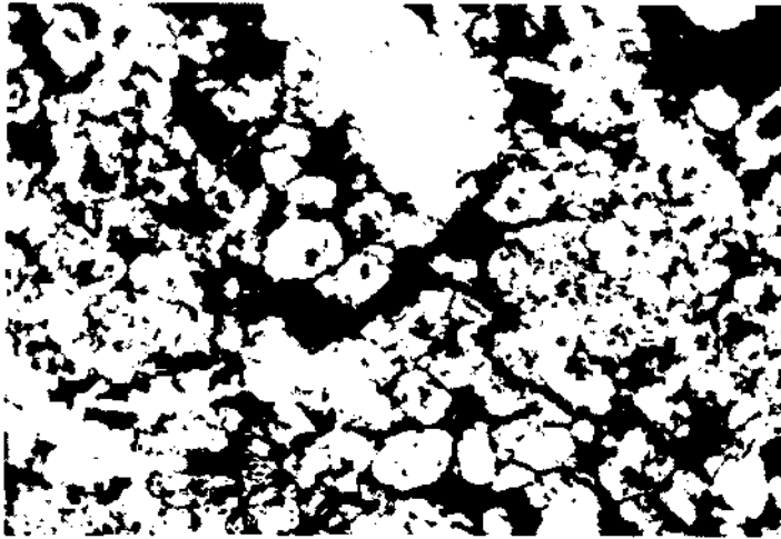
Foto 21 - Okular: 10, Objektiv: 16, in der Luft. Die Lagerstätte von Siirt-Madenköy. Magnetit (grau) tritt in Form von rundlichen Gebilden auf und zwischen ihnen befinden sich Pyrit (weiss) und Gang (schwarz).
