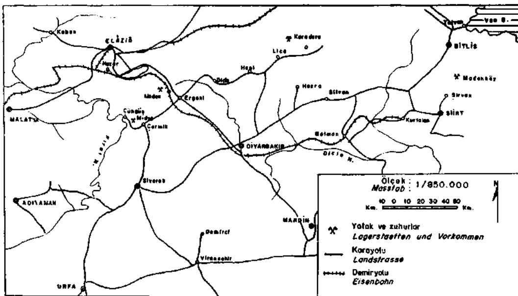
Abb. 1 - Lokationskarte der Kupfererzlagerstaetten und -vorkommen in Südostanatolien.
