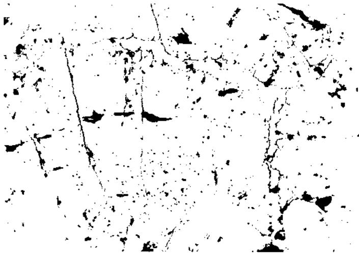
Foto 3 - Okular: 10, Objektiv: 25, im Immersionsöl. Das Kisa Bekir-Vorkommen in Ergani Maden. Kataklastische Risse des Pyrits (hellstgrau) sind mit Kupferkies (hellgrau) gefüllt. Löcher und Gang (schwarz).
