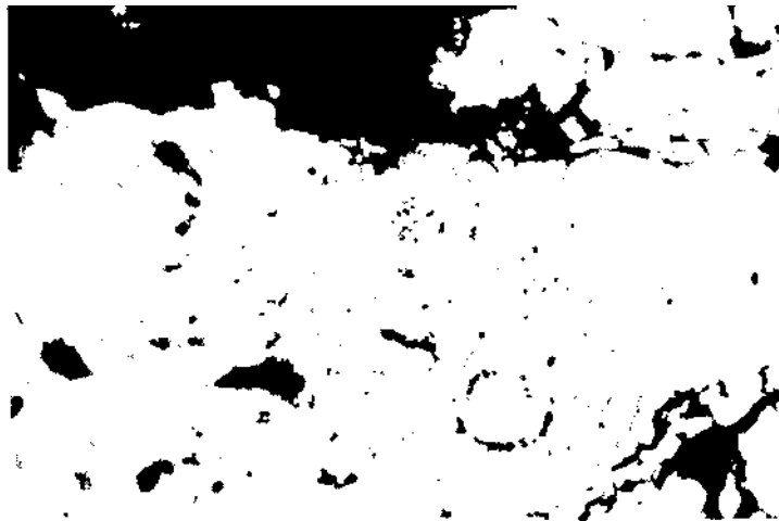
Foto 4 - Okular: 10, Objektiv: 60, im Immersionsöl. Das Kisa Bekir-Vorkommen in Ergani Maden. Pyrit (von lichterer Farbe und Relief aufweisend) zeigt mit Kupferkies (hellgrau und vorherrschend) kolloidale Verwachsung. Gangmineral Chlorit und Löcher (schwarz).
