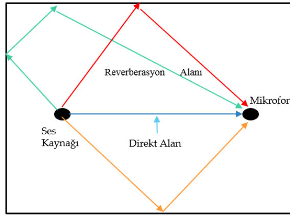
Şekil 2. Sesin Oda İçinde Yansıması
