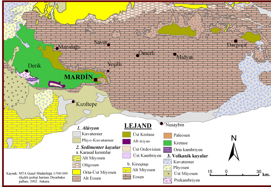
Şekil. 1. Midyat ve çevresi jeoloji haritası
