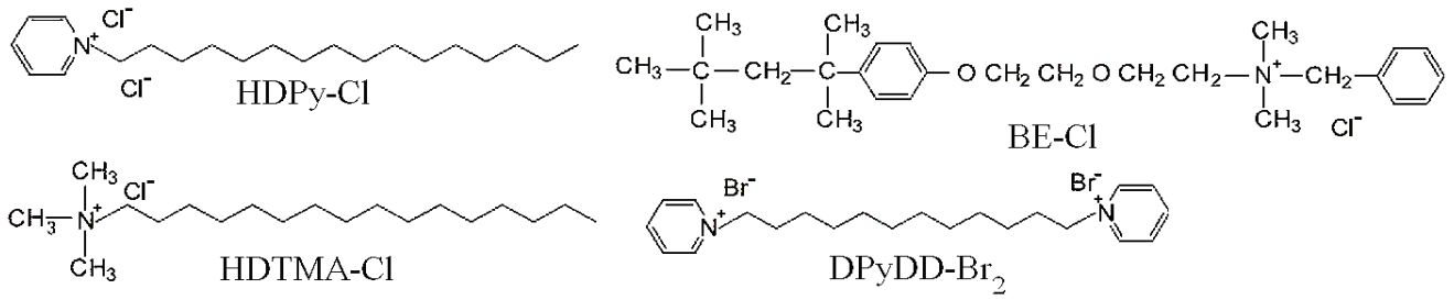
Şekil 1. Bazı organik YAM bileşikler ([46]'dan uyarlanmıştır)
