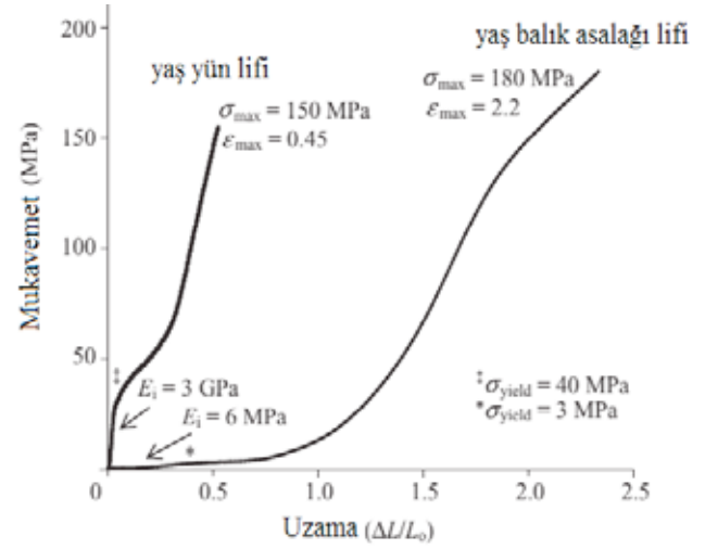
Şekil 4. Balık asalağı salgı lifleri (yaş) ile yün liflerinin (yaş) mukavemet-uzama eğrilerinin karşılaştırılması [36]
