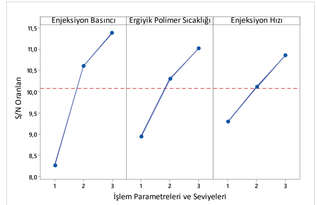
Şekil 7. % incelleme oranları için ortalama S/N grafiği (Daha büyük daha iyi)
