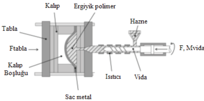
Şekil 1. Plastik enjeksiyon kalıplama yöntemi ile sac şekillendirme
