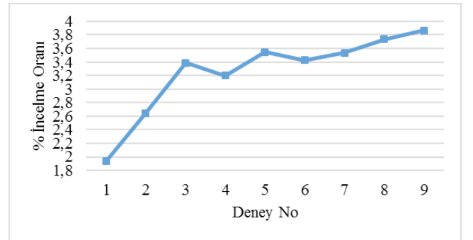
Şekil 6. 1,5 mm kalınlığına sahip alüminyum plakaların A-A ve B-B kesitleri boyunca meydana gelen % incelleme değişimleri
