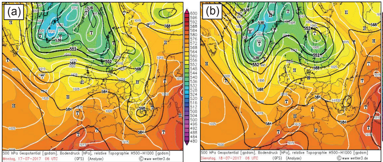
Şekil 3. Yer ve yukarı seviye haritalarının (a) 17 Temmuz 2017 06:00 UTC ve (b) 18 Temmuz 2017 06:00 UTC harita analizleri
