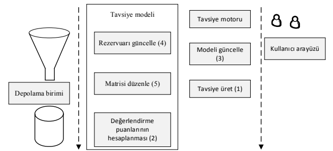
Şekil 2. TeRec mimarisi
