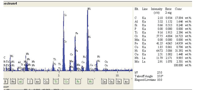
Şekil 15. EDS analiz görüntüsü (x500)
