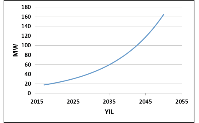
Şekil 8: Keşan ilçesi'nde 2050 yılına kadar gerekli kurulu rüzgar gücünün değişimi
