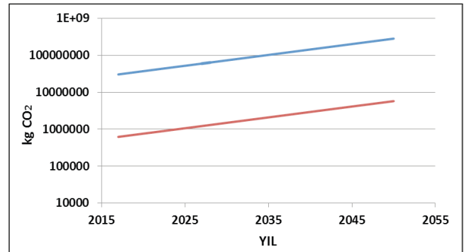
Şekil 9: Keşan ilçesi'nde mevcut kaynaklar ve rüzgar ile elektrik üretimi ile CO 2 salınım değişimleri. Mavi: Mevcut kaynaklar; Kırmızı: Rüzgar
