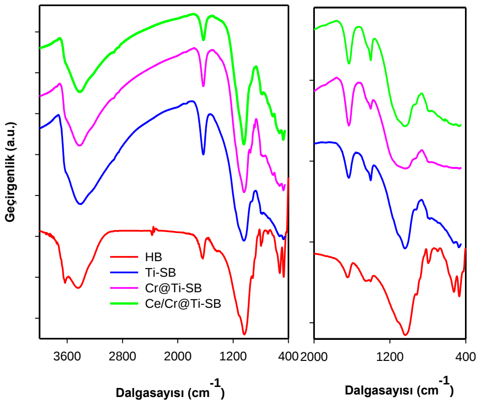
Şekil 4. HB ve sütunlu kil örneklerinin (a) amonyak adsorpsiyonundan önce 400\text{-}4000\text{ cm}^{-1} dalga sayısı aralığındaki (b) amonyak adsorpsiyonundan sonra 400\text{-}2000\text{ cm}^{-1} dalga sayısı aralığındaki FTIR grafikleri
