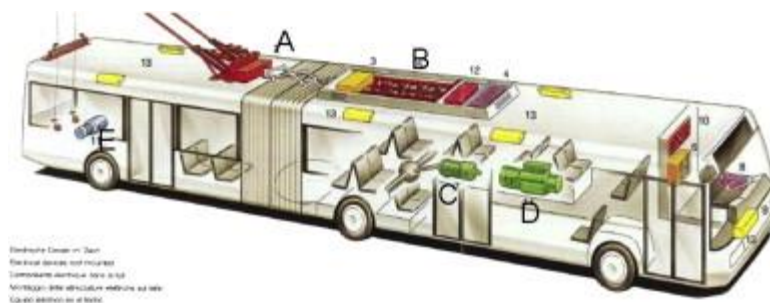
Şekil 2. Modern trolleybüs için konsept araç tasarımı (Kühne, 2010)
