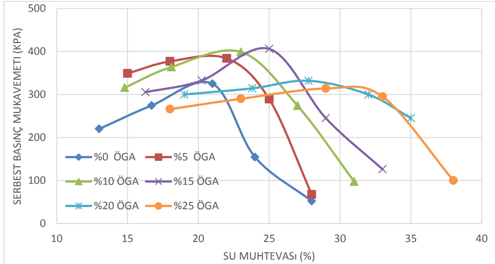
Şekil 6. CL-ÖGA numunelerinin su muhtevasına bağlı serbest basınç dayanımı
