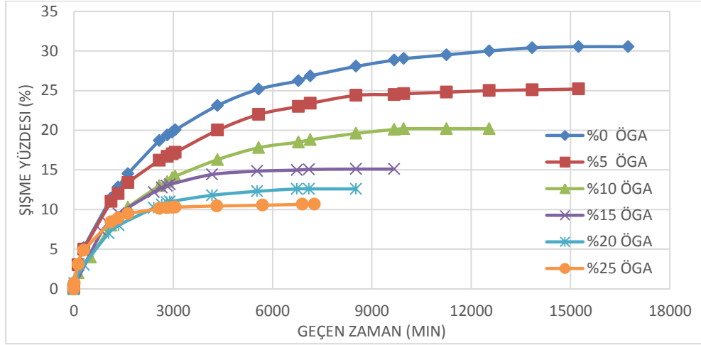
Şekil 8. CH-ÖGA numunelerinin zamana bağlı olarak şişme yüzdeleri
