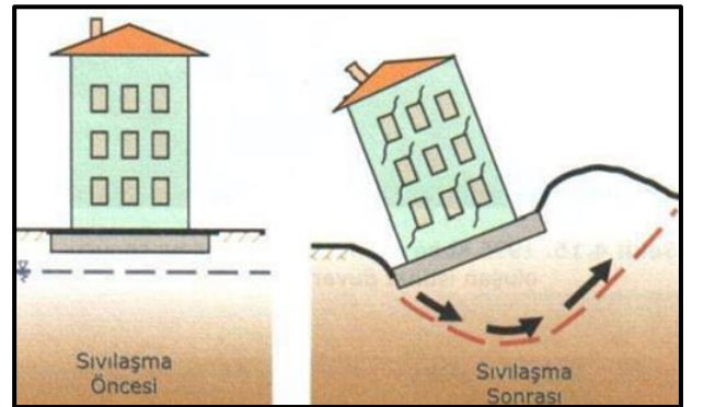
Şekil 13. Taşıma gücü kaybı nedeniyle oluşan göçme (Çıklaiblikçi, 2019)
