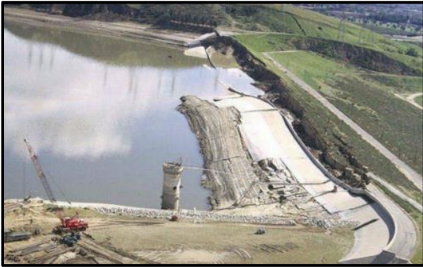
Şekil 2. San Fernando (1971) depreminde sıvılaşma sonucu oluşan hasarlar (Koçkar, 2022)
