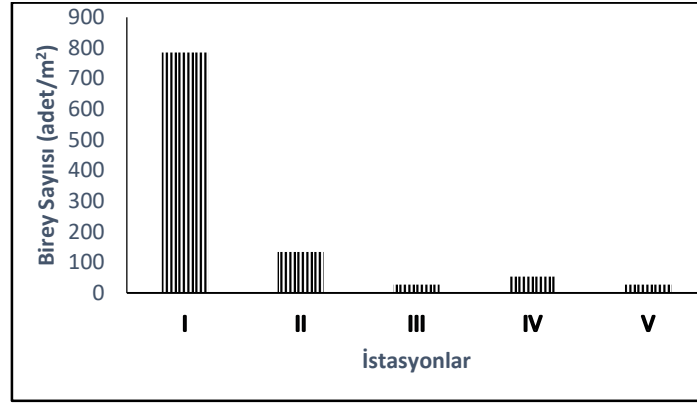
řekil 2. Deęirmen deresinde bentik makroomurgasızların toplam bolluklarının deęiřimi (adet/m²)
