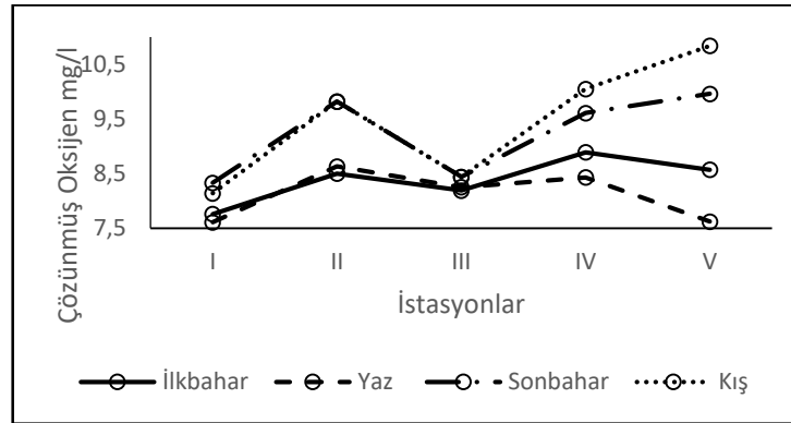
Şekil 5. Değirmen deresinde ortalama çözülmüş oksijen değerinin mevsimlere ve istasyonlara göre değişimi (mg/l)
