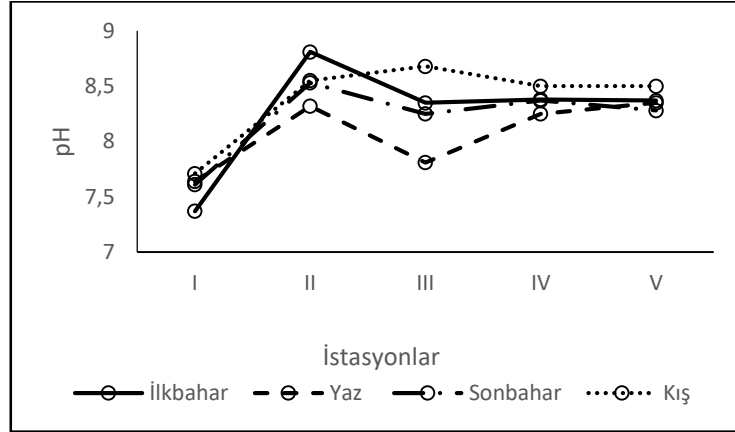
Şekil 7. Değirmen deresinde ortalama pH değerinin mevsimlere ve istasyonlara göre değişimi
