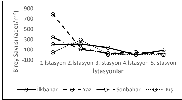
řekil 3. Deęirmen deresinde bentik makroomurgasızların mevsimlere gre istasyonlardaki deęiřimi (adet/m²)
