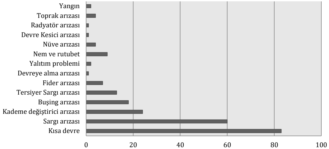
Şekil 1. Güç transformator arızalar
