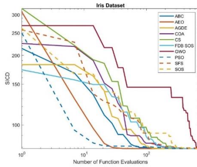
(a) Iris Veri Seti (Iris Dataset)
