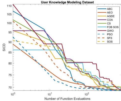
(d) User Knowledge Modeling Veri Seti (User Knowledge Modeling Dataset)
