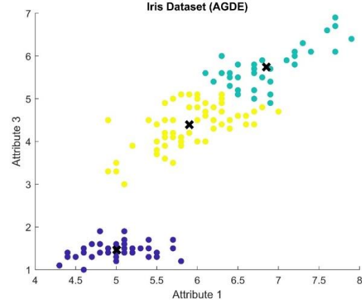
(b) Iris Veri Seti (Iris Dataset)
