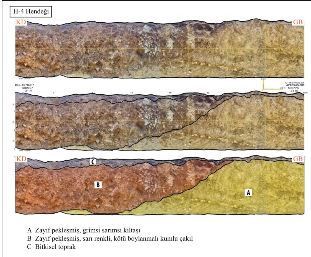
Şekil 12. H-4 Hendeginin GD Duvarının Fotomozayığı İle Yorumlanmış Log Görünümü (Log View Of The SE Wall Of Trench H-4 İnterpreted With Photomosaic)
