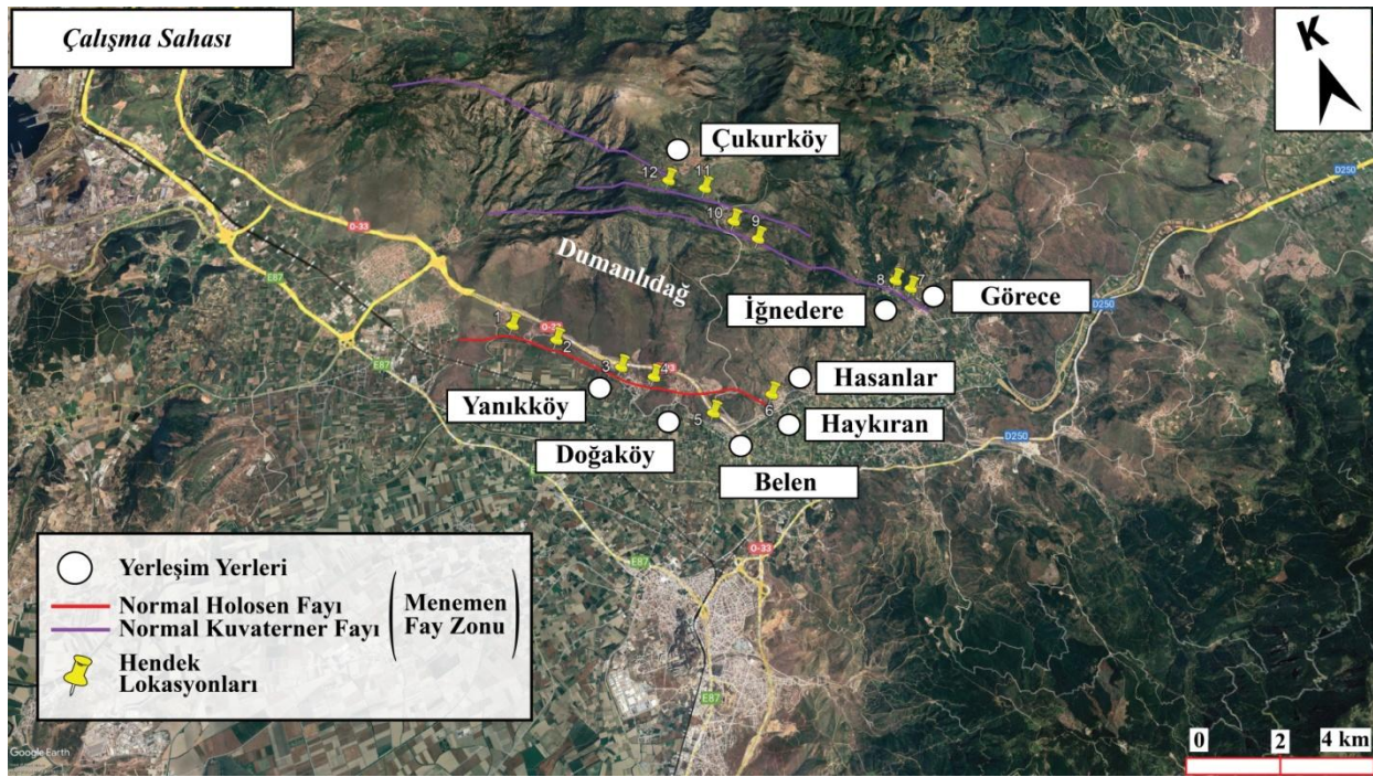
Şekil 1. Çalışma Sahası Çevresini Ve Gerçekleştirilen Çalışmalara Ait Lokasyonları Gösterir Harita (Map Showing The Surroundings Of The Work Area And The Locations Of The Work Carried Out.)
