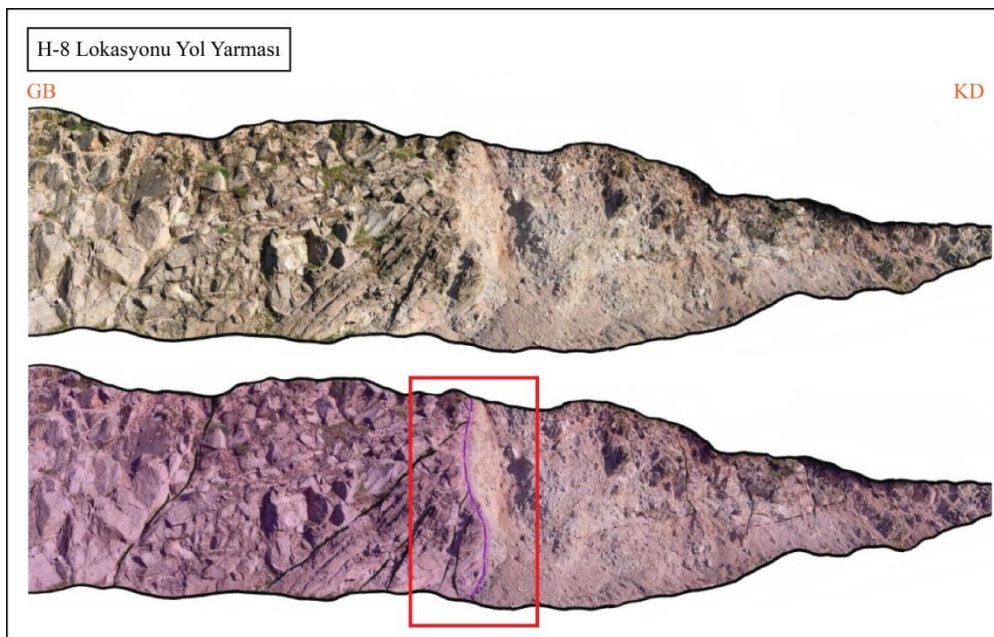
Şekil 17. H-8 Hendeğinin GD Duvarının Fotomozayiği İle Log Görünümü (Log View With Photomosaic Of The SE Wall Of Trench H-8)
