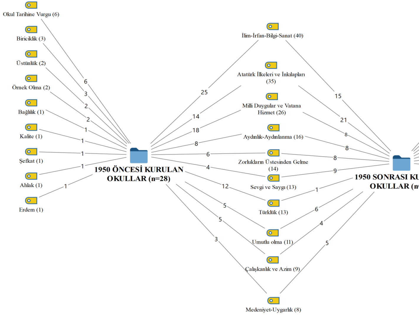
Şekil 12. 1950 Öncesi ve Sonrası Kurulan Okulların Marşlarında Yer Alan Değerlerin İkili Vaka Modeli
