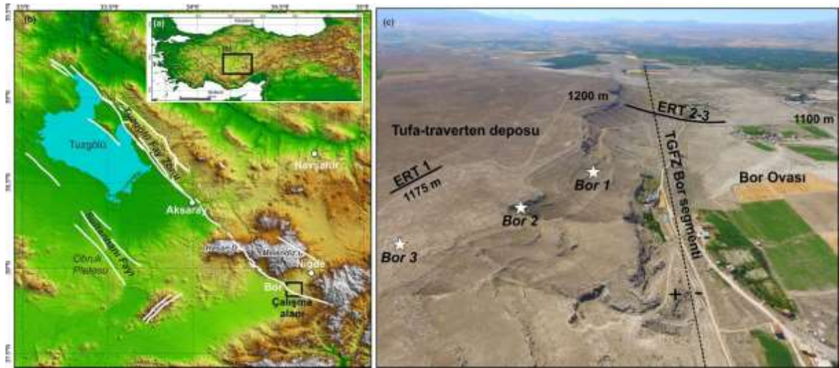
Şekil 1: (a, b) Tuzgölü Fay Zonu [9] ve (c) deponun havadan görünümü, örneklem ve ölçüm yapılan alanları
