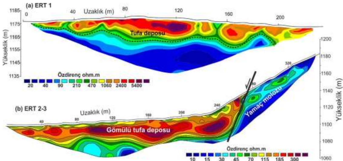
Şekil 2: (a) Deponun üstünden (ERT1) ve (b) güney yamacından yapılan (ERT2-3) ERT profil çözümlemeleri
