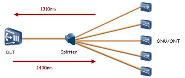
Şekil 4. Basit GPON çalışma prensibi [6].
