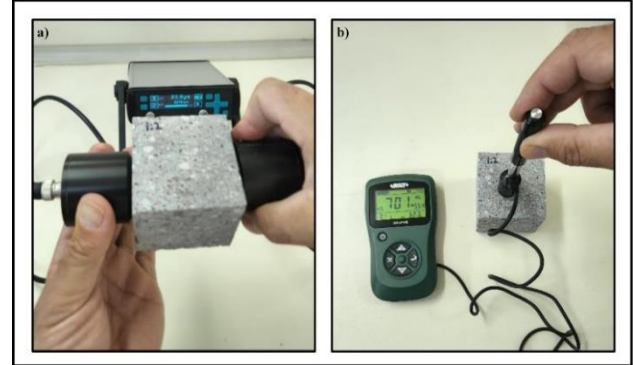
Şekil 3. Kayaçlarda bazı fiziksel özelliklerin ölçümü: (a) P-dalgası hızı, (b) Leeb sertliği
