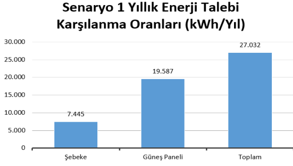
Şekil 6. Senaryo 1’deki yıllık enerji talebi karşılama oranları
