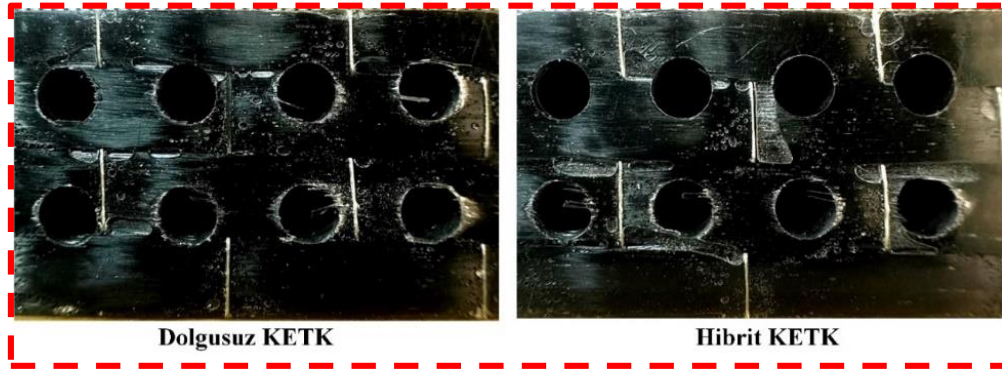
Şekil 9. Dolguşuz ve hibrit KETK'lerin delik delme sonrası delaminasyon görüntüleri
