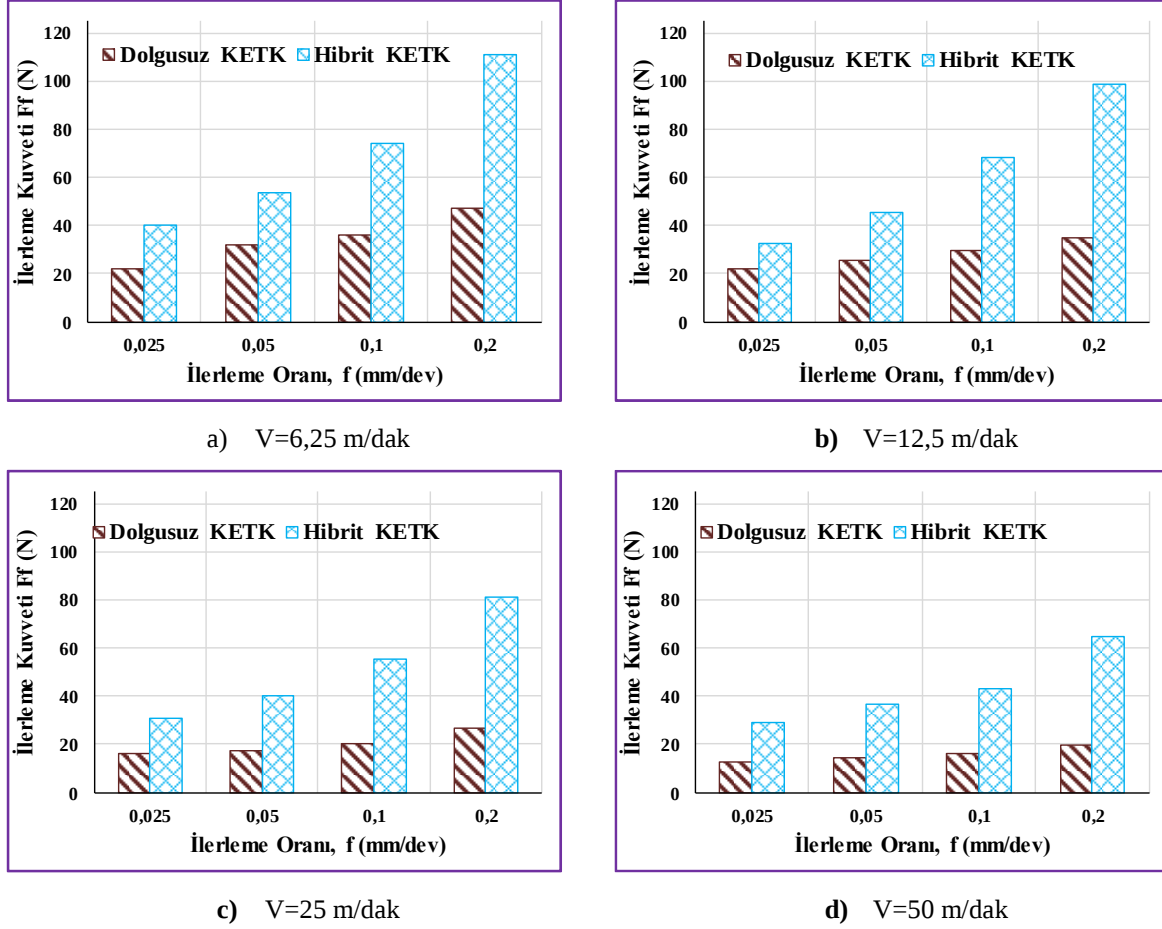
Şekil 6. Dolgunuz ve hibrit KETK'lerin farklı kesme hızlarında elde edilen ilerleme kuvvetleri değerleri
