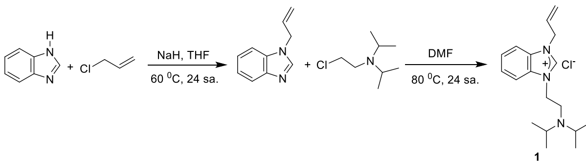
Şekil 1. 1-Allil-3-(2-diizopropilaminoetil)benzimidazolyum klorür'ün (1) sentezi
