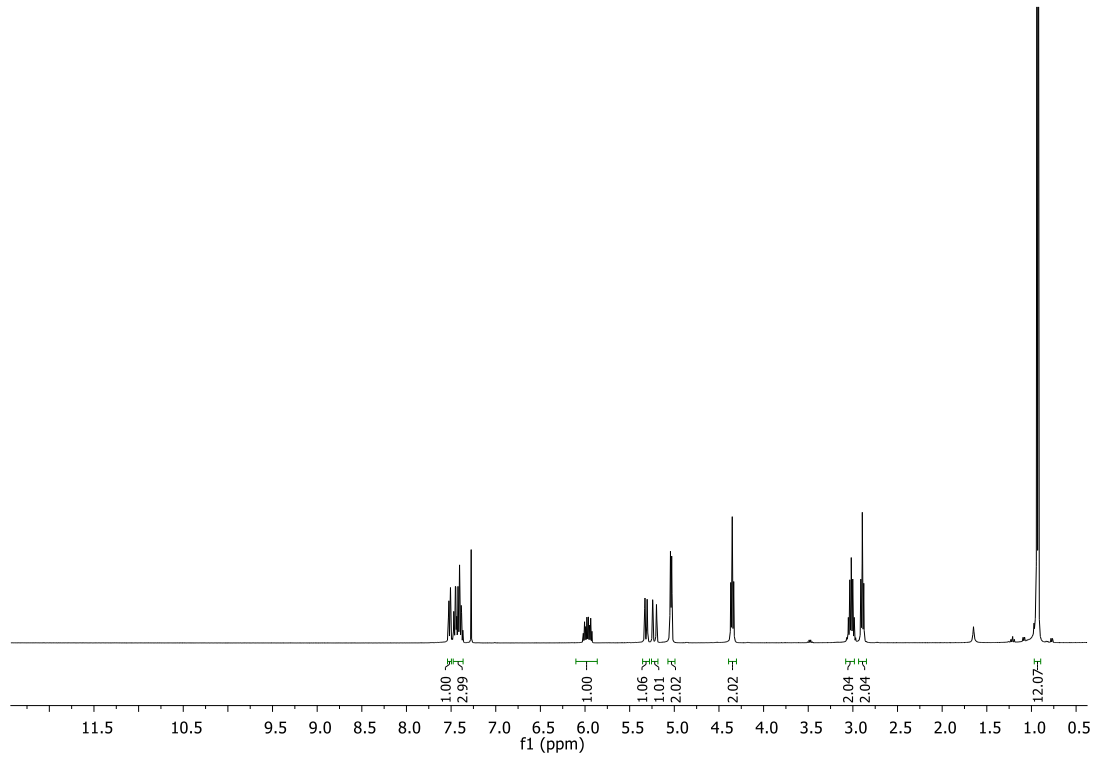
Şekil 7. 2 Bileşiğine ait 1 H NMR spektrumu
