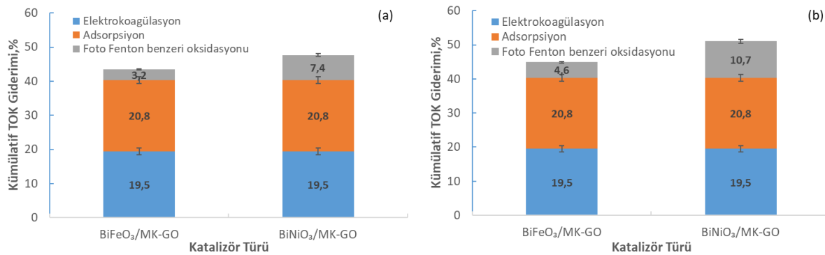
Şekil 9. Hibrit Arıtım Sisteminin Foto Fenton Benzeri Oksidasyonu Adımında 0,25 g/L (a) ve 0,5 g/L (b) Katalizör Kullanılarak Elde Edilen TOK Giderimi
