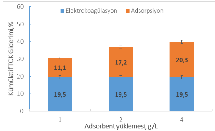
Şekil 6. Hibrit Arıtım Sisteminin Adsorpsiyon Adımında Adsorbent Yüklemeinin TOK Giderimi Üzerine Etkisi
