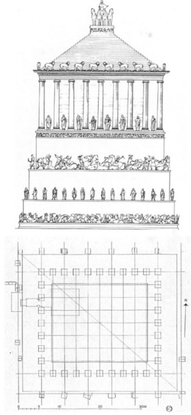
Şekil 1. Maussoleion plan ve rekonstrüksiyon önerisi (Jeppesen, 1992: taf. 21. 1-2).
