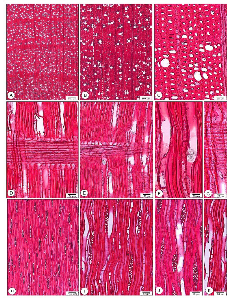
Şekil 2. Anadolu şimşiri gövde odununun enine, radyal ve teğet kesitlerine ait mikrofotograflar Figure 2. Microphotographs of transverse, radial and tangential sections of Anatolian boxwood stem wood
