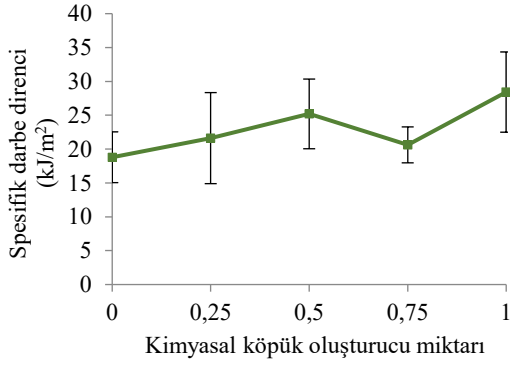
Şekil 2. PVC köpüklerin spesifik darbe direnci grafiğı Figure 2. Specific impact strength graph of PVC foams
