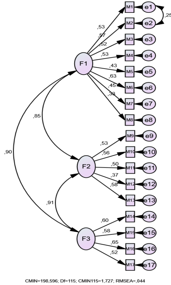
Şekil 1. Doğrulayıcı Faktör Analizi Yol Şeması
