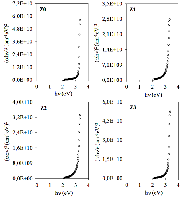
Şekil 3. ZnO filmlerinin (\alpha h\nu)^2 \sim h\nu değişim grafikleri
