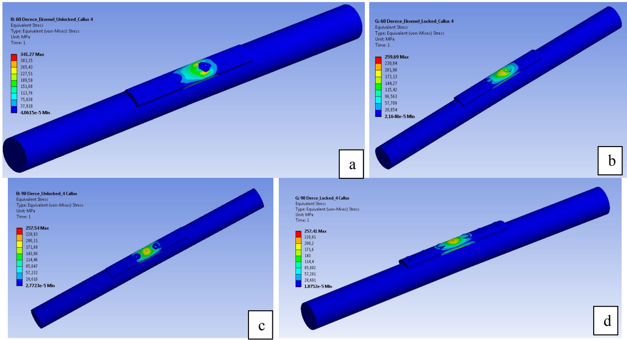
Şekil 4. Kemik-kallus-implant toplam modellerinde oluşan gerilmeler; (a) 60° kırık kilitli plak, (b) 60° kırık kilitli plak, (c) 90° kırık kilitli plak ve (d) 90° kırık kilitli plak
