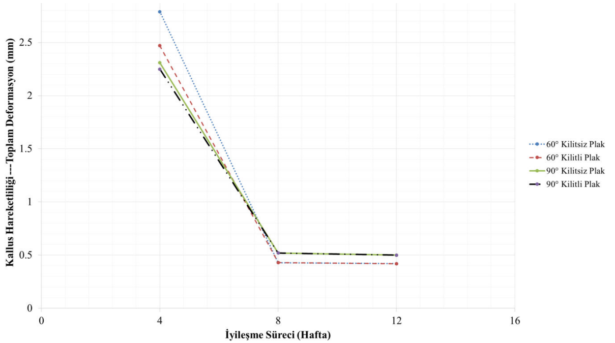
Şekil 8. Kallus mekanik özelliklerinin iyileşme sürecindeki etkisi
