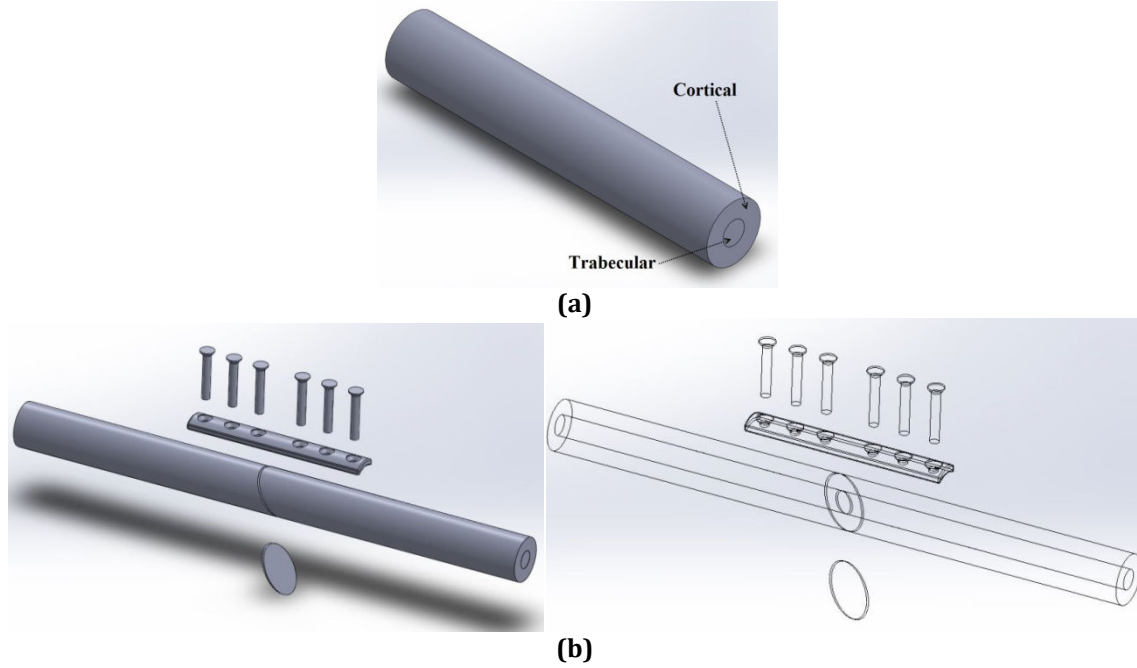
Şekil 2. 3B modeller. (a) Kortikal ve trabeküler olarak ayrılmış tibia modeli, (b) kamık-plak-vida-callus yapılarının yerleşimi
