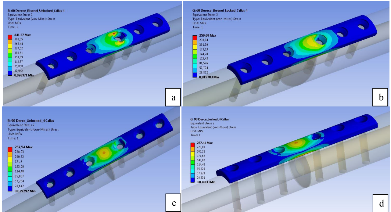
Şekil 5. Plak modellerinde oluşan gerilmeler; (a) 60° kırık kilitli plak, (b) 60° kırık kilitli plak, (c) 90° kırık kilitli plak ve (d) 90° kırık kilitli plak
