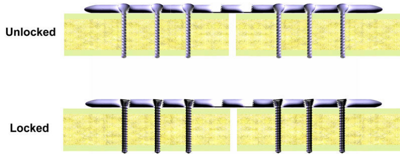
Şekil 1. Kilitli ve kilsiz plak sistemlerinin şematik gösterimi (Gardner vd. 2006)
