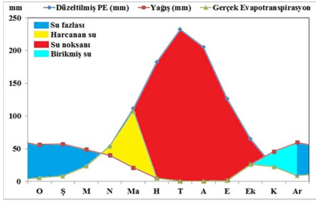
Şekil 2. Gölarmara'nın su bilançosu.
