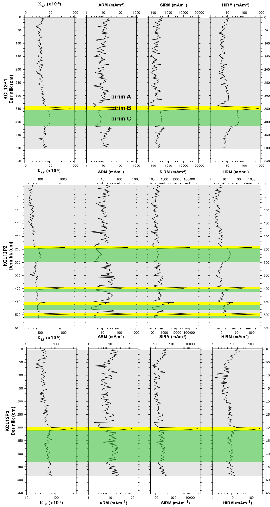
Şekil 2. KCL12P1-P2-P3 karotlarının derinlik boyunca \kappa_{LF} (Makaroğlu, 2021), ARM, SIRM ve HIRM değişimlerini içeren manyetik mineral yoğunluğu.
