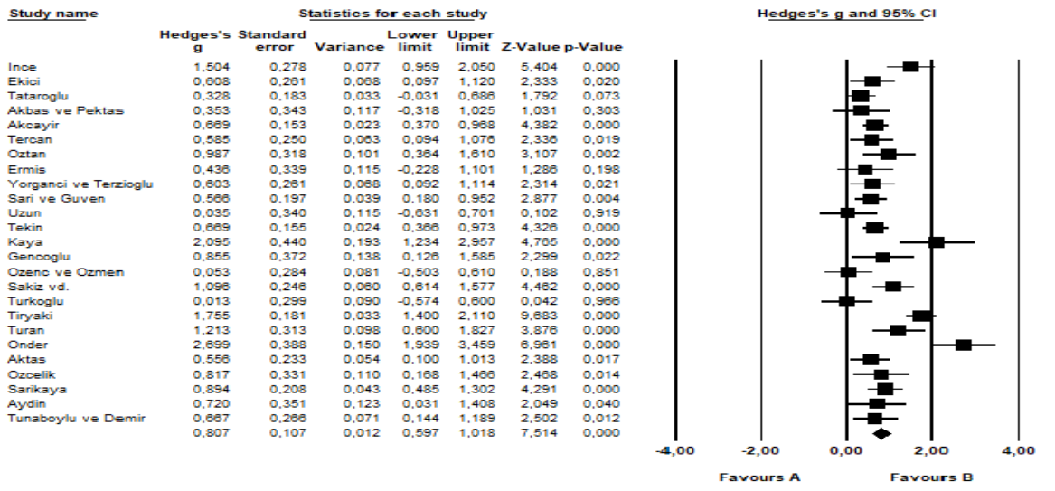
Şekil 2. Rastgele etkiler modeline göre çalışmaların etki büyüklüklerine ait grafiği
