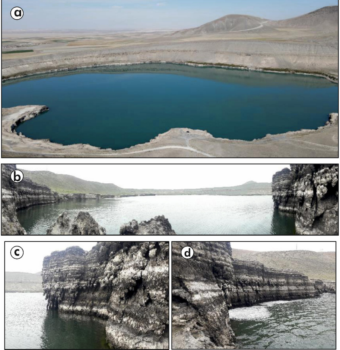
Fotoğraf 3: a) Acıgöl'ün Güneybatı Yönünden Genel Görünümü ve Gerisindeki Karacadağ Kütlesi, b) Acıgöl'ün Maar Tabanından Gölün Görüntüsü, c-d) Acıgöl'de Su Seviyesinin Düşmesinden Sonra Kıyılarda Ortaya Çıkan Diklikler ve Su Kimyasının Bunlar Üzerindeki Etkisi
