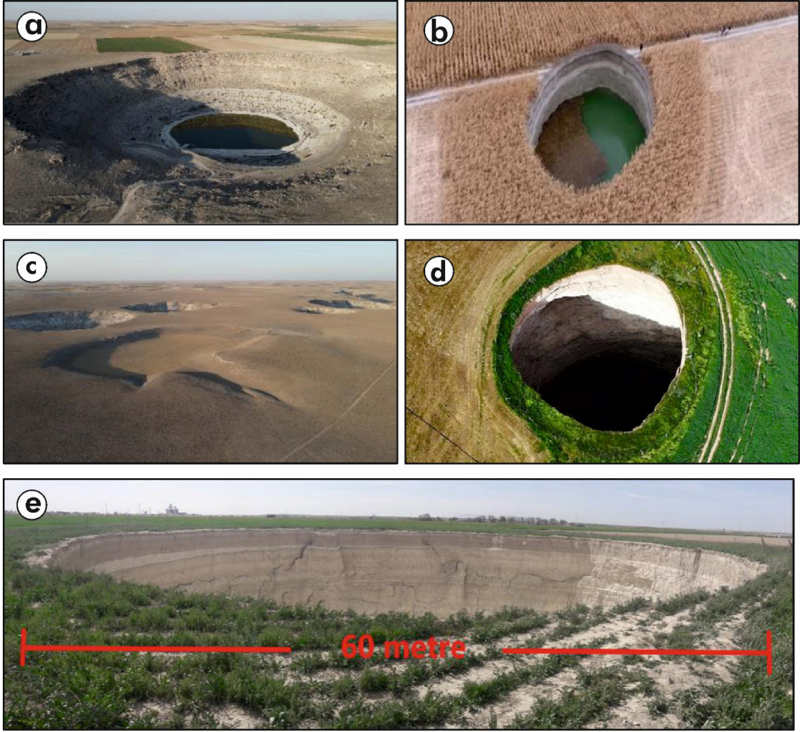
Fotoğraf 5: a) Meyil Obruğu b-c-d) Obruk Platosu Üzerinde Bulunan Çeşitli Obruklar e) Yarımoğlu Obruğu
