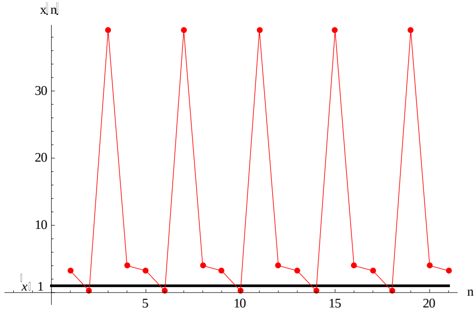
Şekil 5. x(n) çözümlerinin grafiği.
